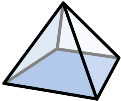
pyramid
