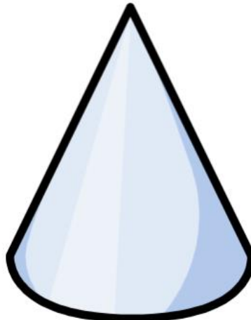
cone
